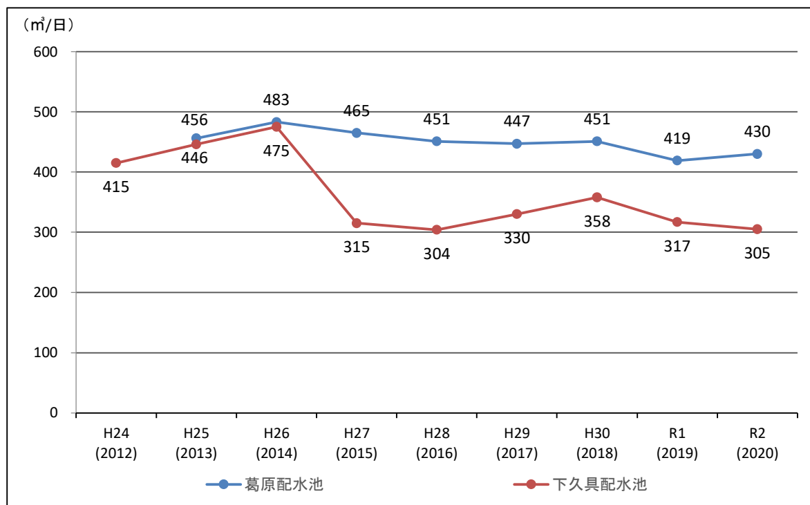
図. 配水池における平均給水量の推移
