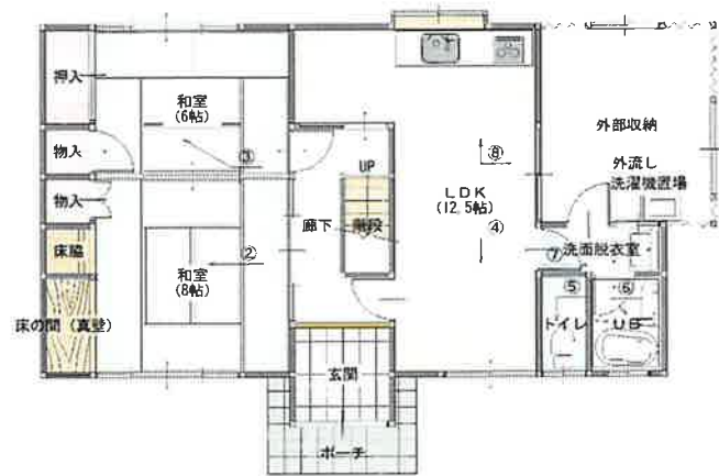
1 階 平面図
